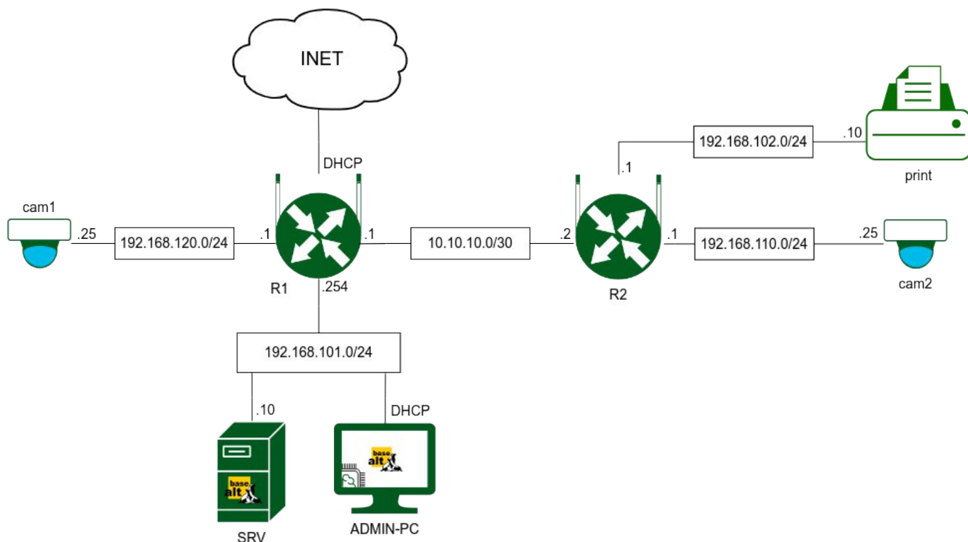
L3 топология
