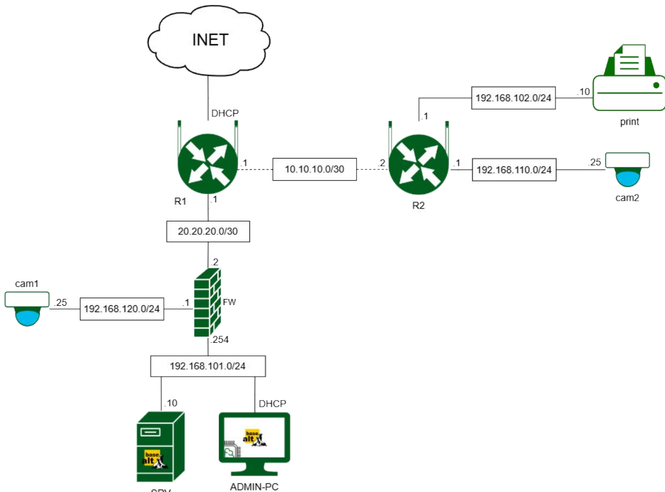
L3 топология
